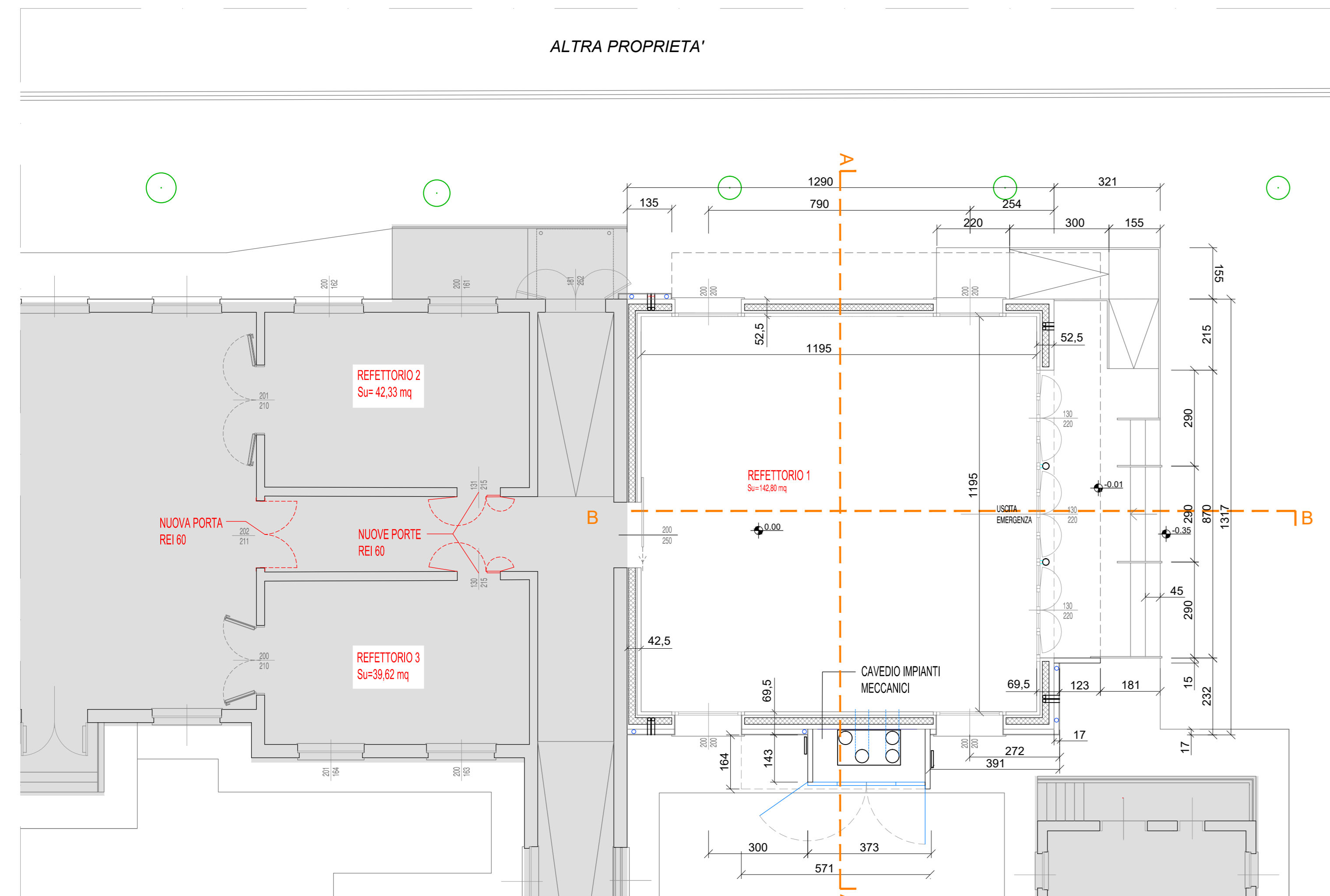
PLANIMETRIA PIANO TERRA CON COLLEGAMENTO A MENSA ESISTENTE scala 1:100
