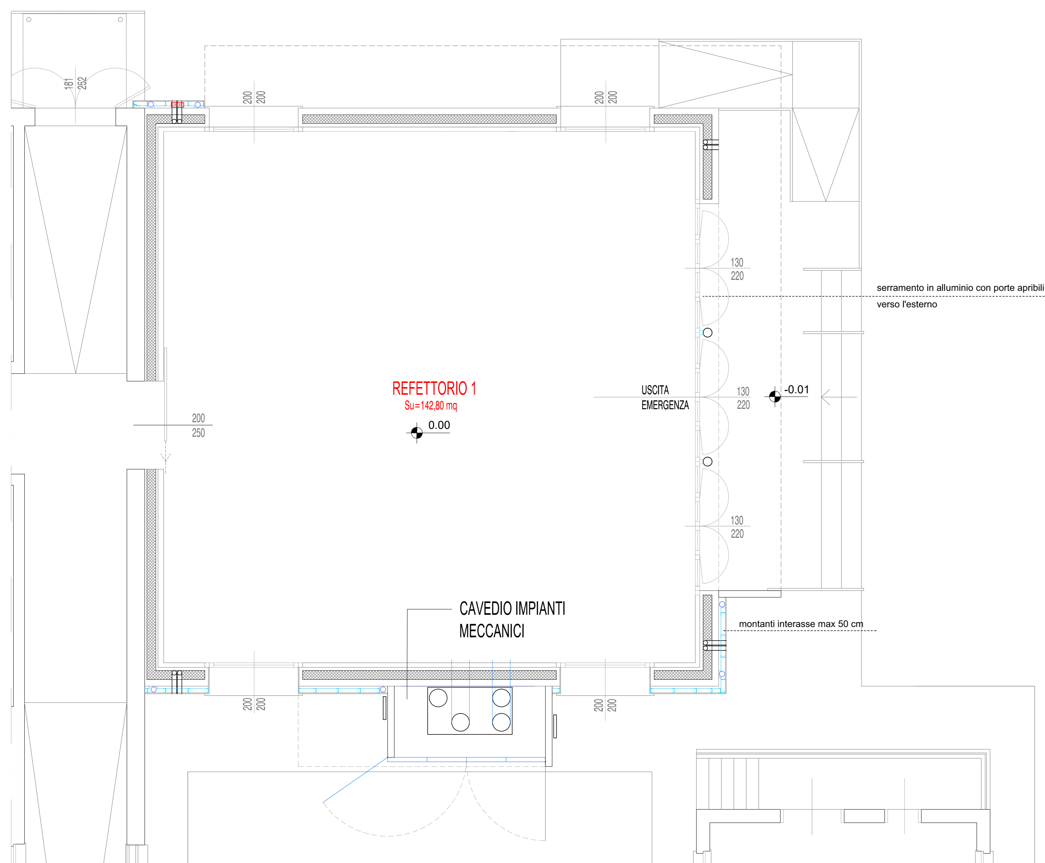
PIANTA INDIVIDUAZIONE MONTANTI A QUOTA +1,10 scala 1:50
