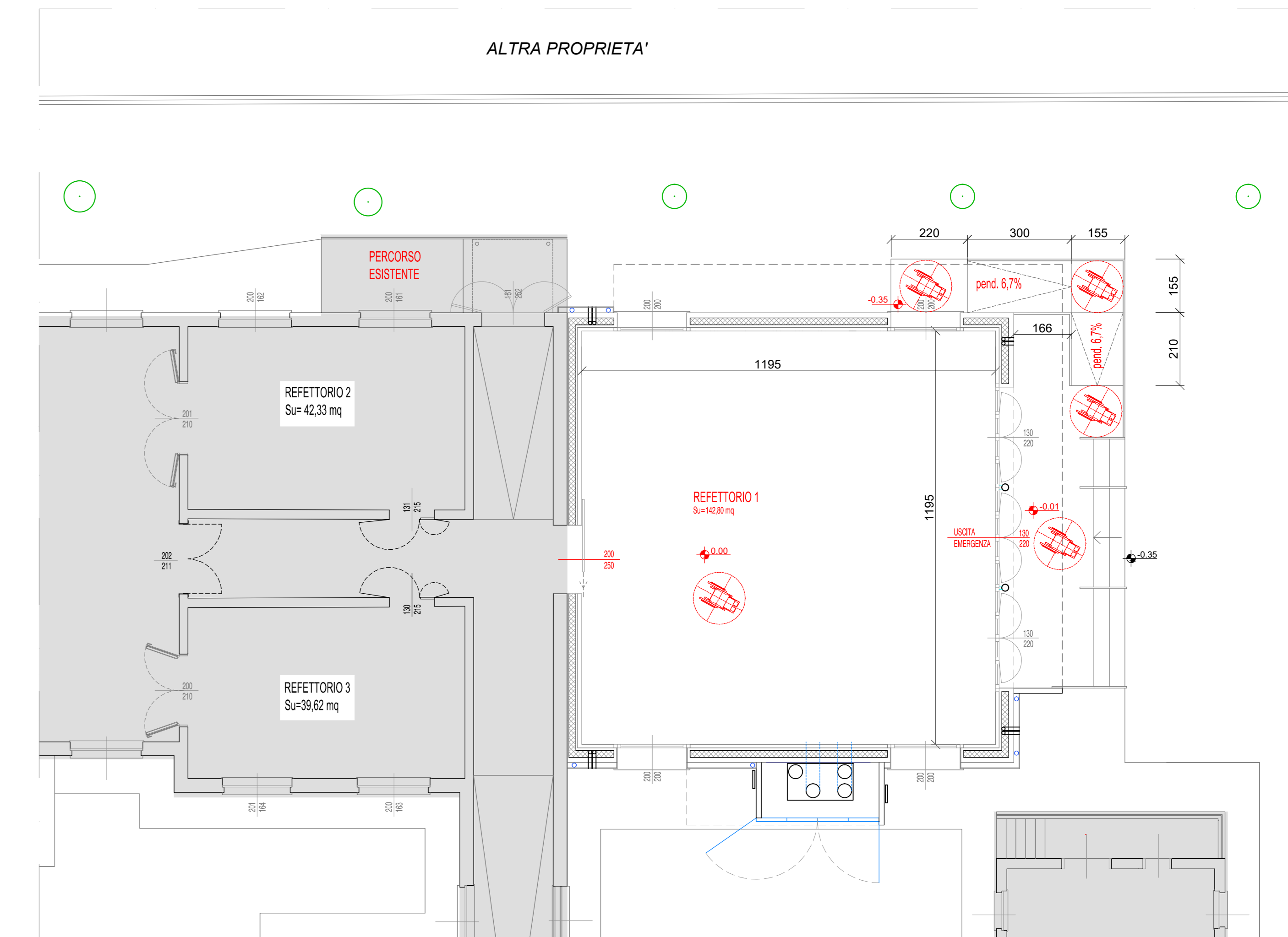
PLANIMETRIA PIANO TERRA VERIFICA ABBATTIMENTO BARRIERE ARCHITETTONICHE scala 1:100
