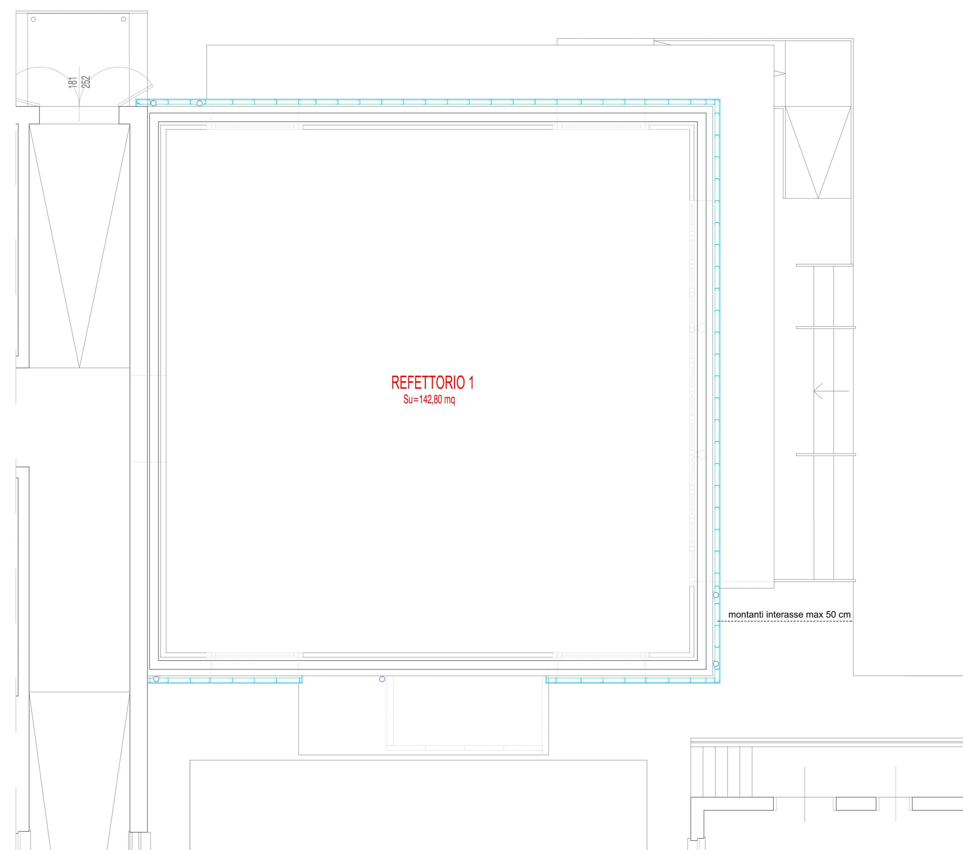
PIANTA INDIVIDUAZIONE MONTANTI A QUOTA +3,90 m scala 1:50
