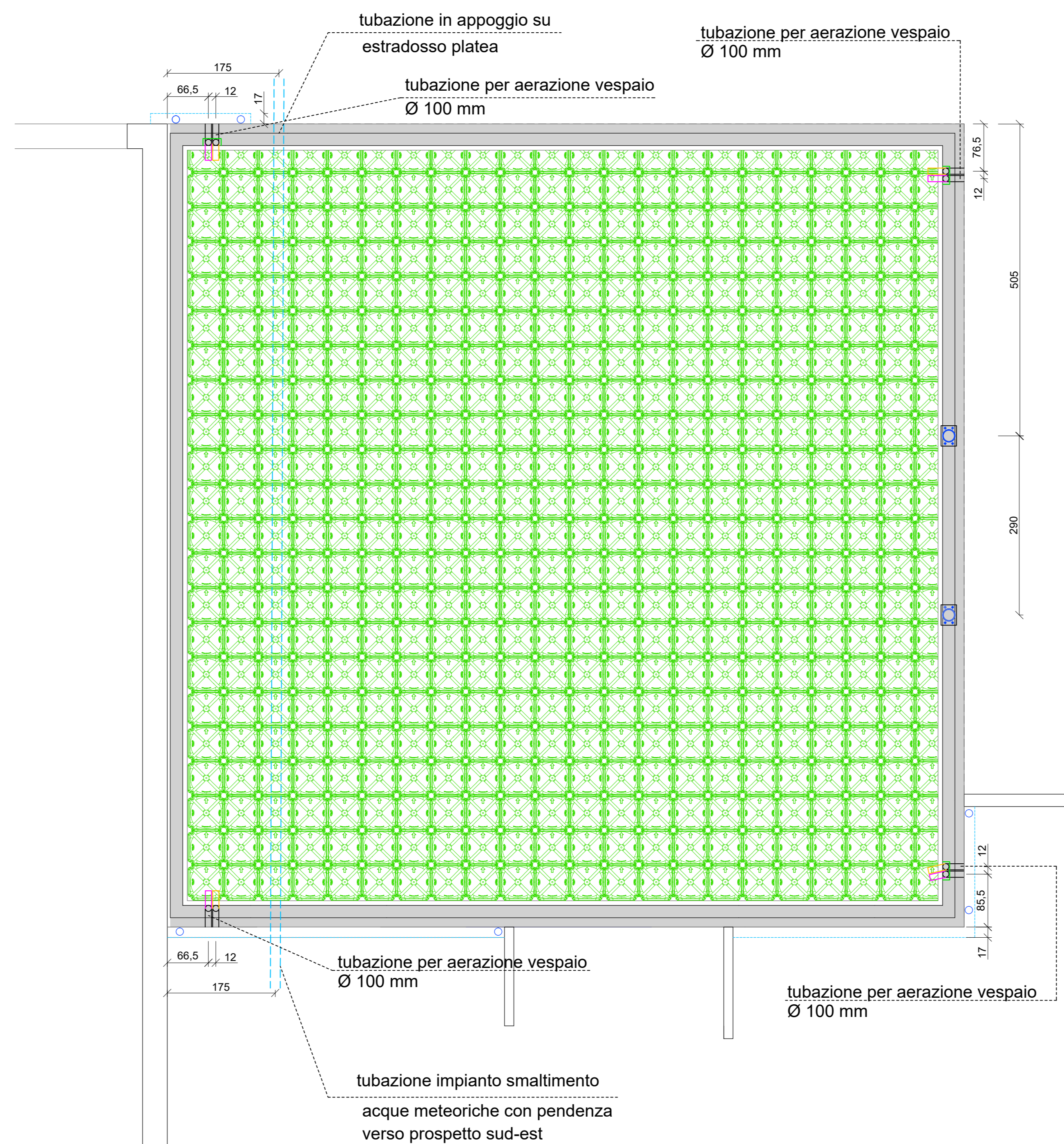
PIANTA VESPAIO AERATO scala 1:50
